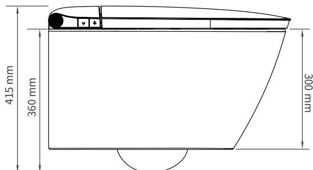
Rysunek miski
